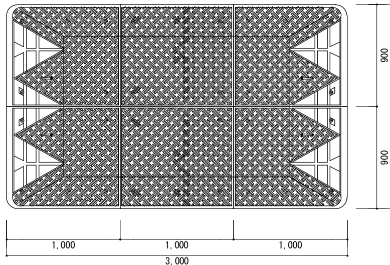
設置例
